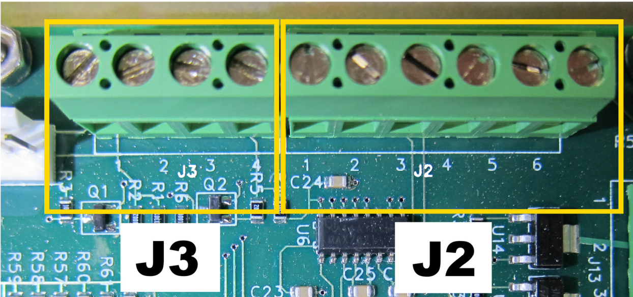
J3 External Encoder (Pulser)
